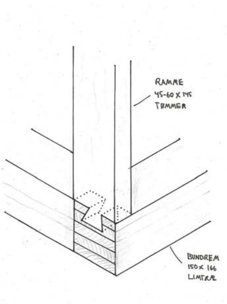
Samling mellem bundrem og ramme med en 'svalehale'
