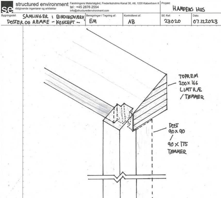
Samling mellem toprem og post med en 'kile' som modvirker træk, hvor remmen kan hvile på posten.
