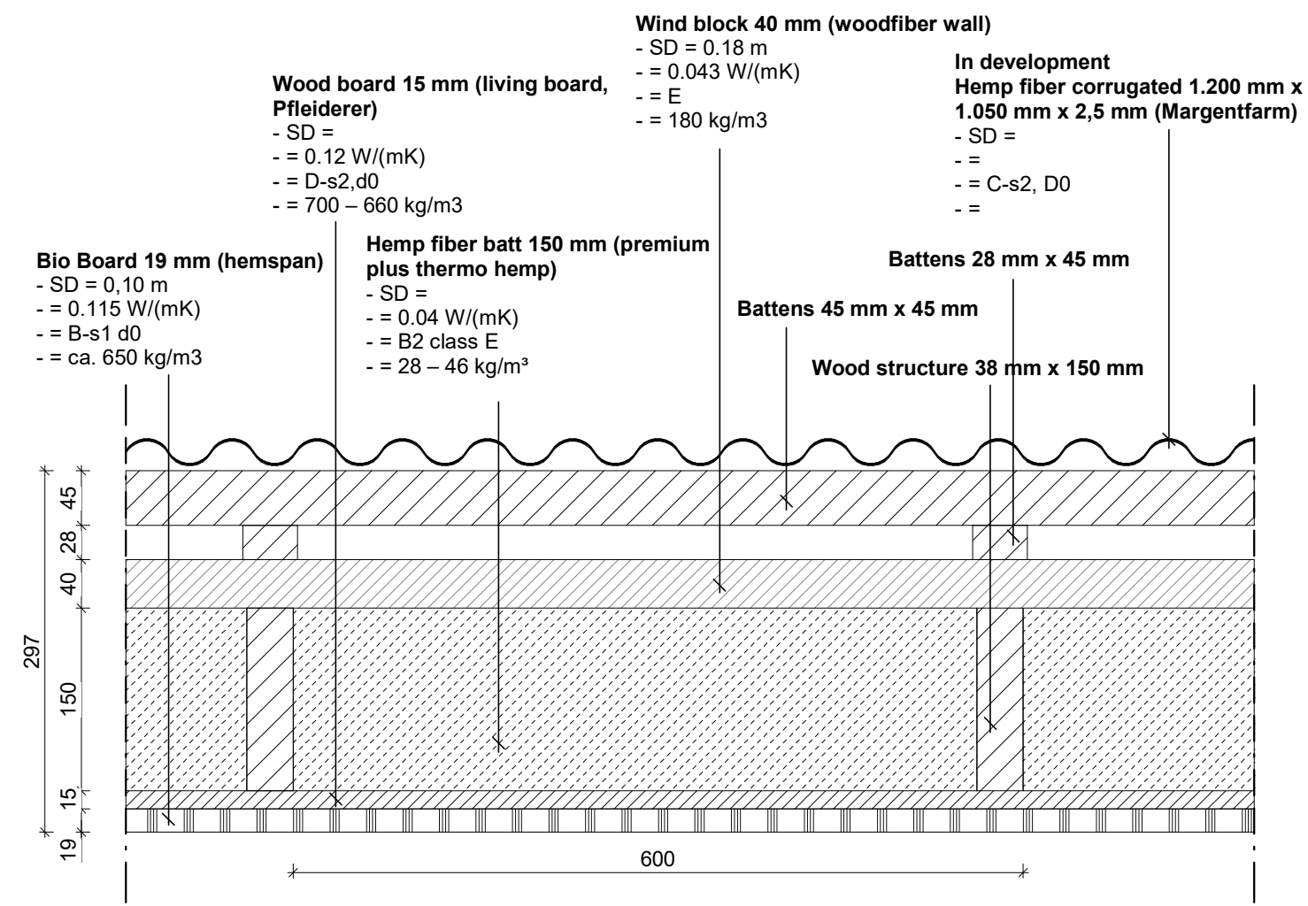
Detail max 15° 1:5
